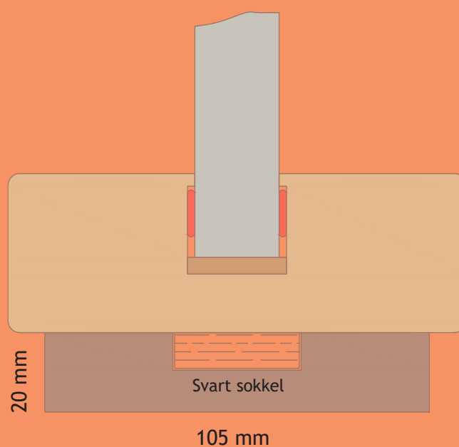
Bunnkarm med inntrukket sokkel sokkel kan utelates om ønskelig
