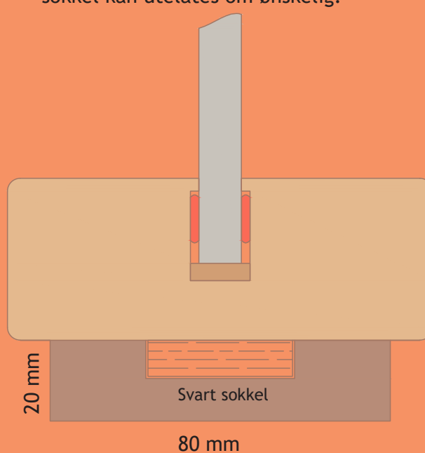
Bunnkarm med inntrukket sokkel sokkel kan utelates om ønskelig.
